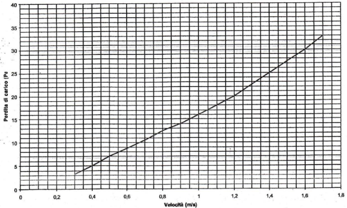
Grafico \Delta p vs. Velocità aria
